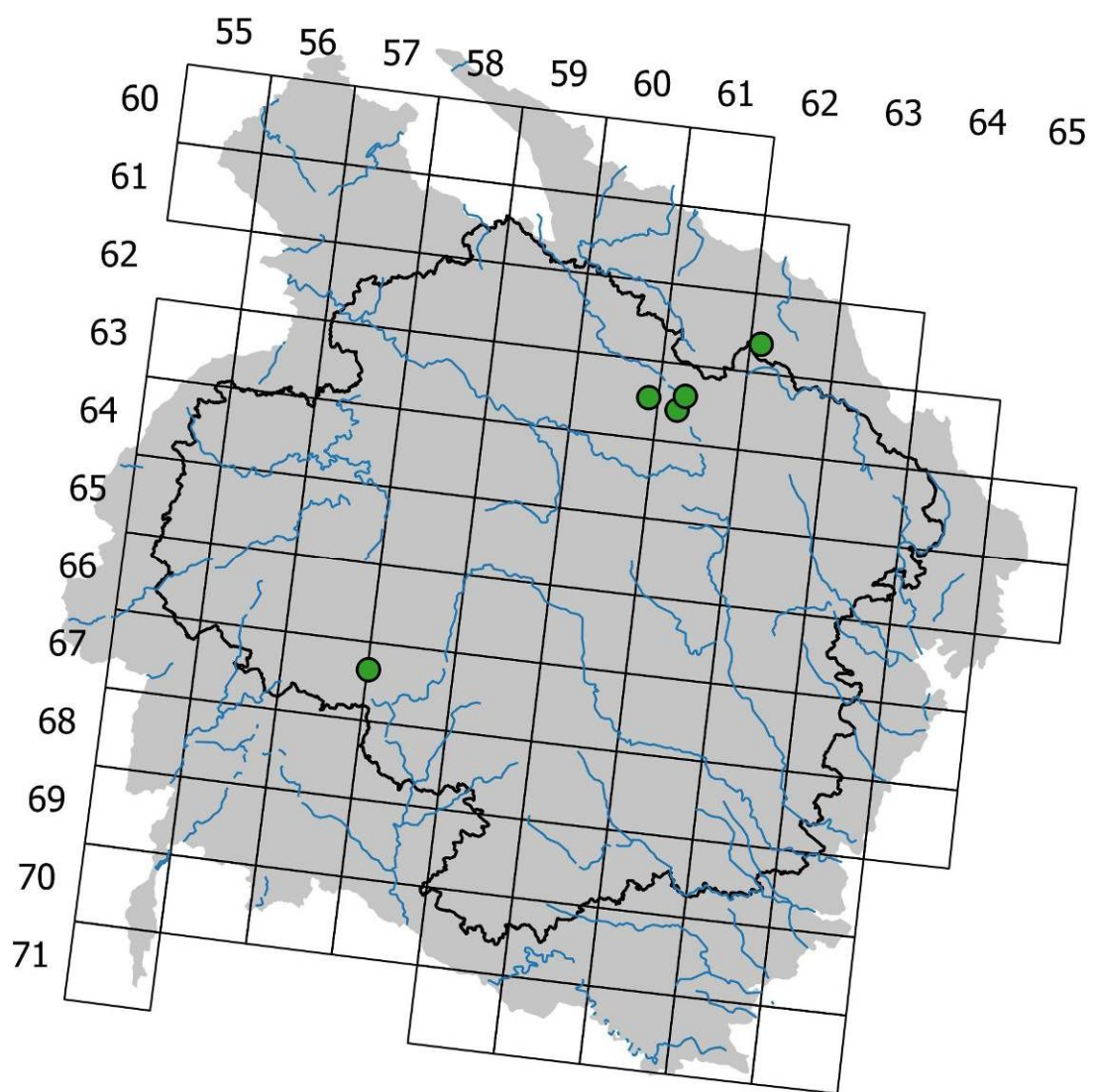
Rozšíření druhu Sphagnum rubellum ; zelený bod – recentní výskyt, černá linie – Kraj Vysočina, modrá linie – řeky, šedivá plocha – Českomoravská vrchovina.
