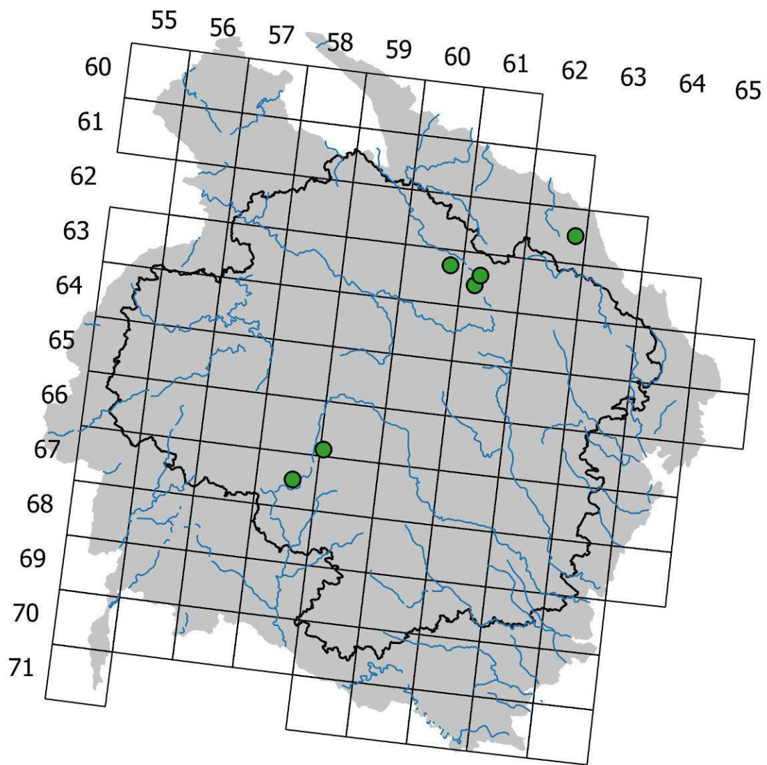
Rozšíření druhu Calypogeia fissa ; zelený bod – recentní výskyt, černá linie – Kraj Vysočina, modrá linie – řeky, šedivá plocha – Českomoravská vrchovina.
